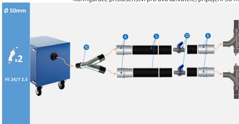
Konfigurace příslušenství pro dva uživatele, připojení 50 mm:
