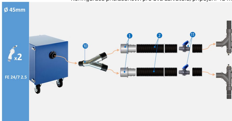
Konfigurace příslušenství pro dva uživatele, připojení 45 mm:
