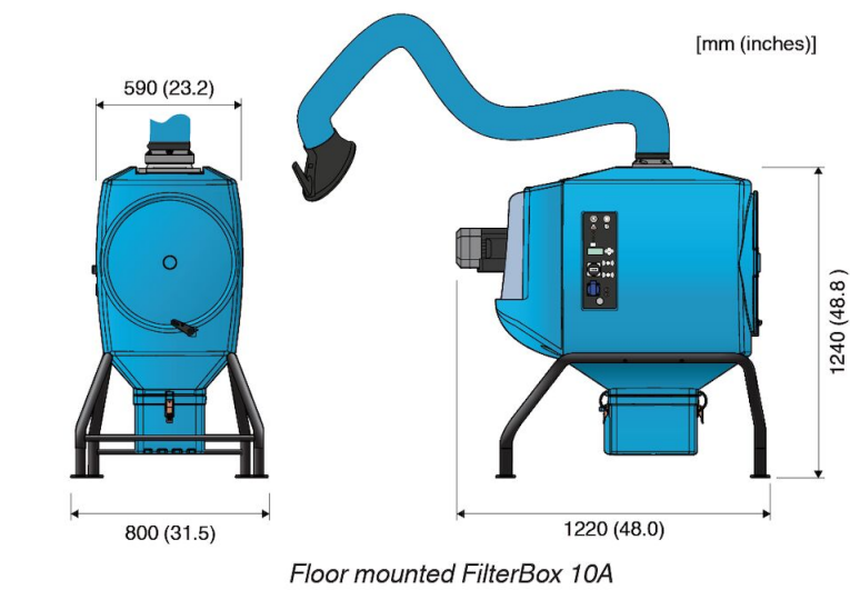
FilterBox 10A Podlahový
