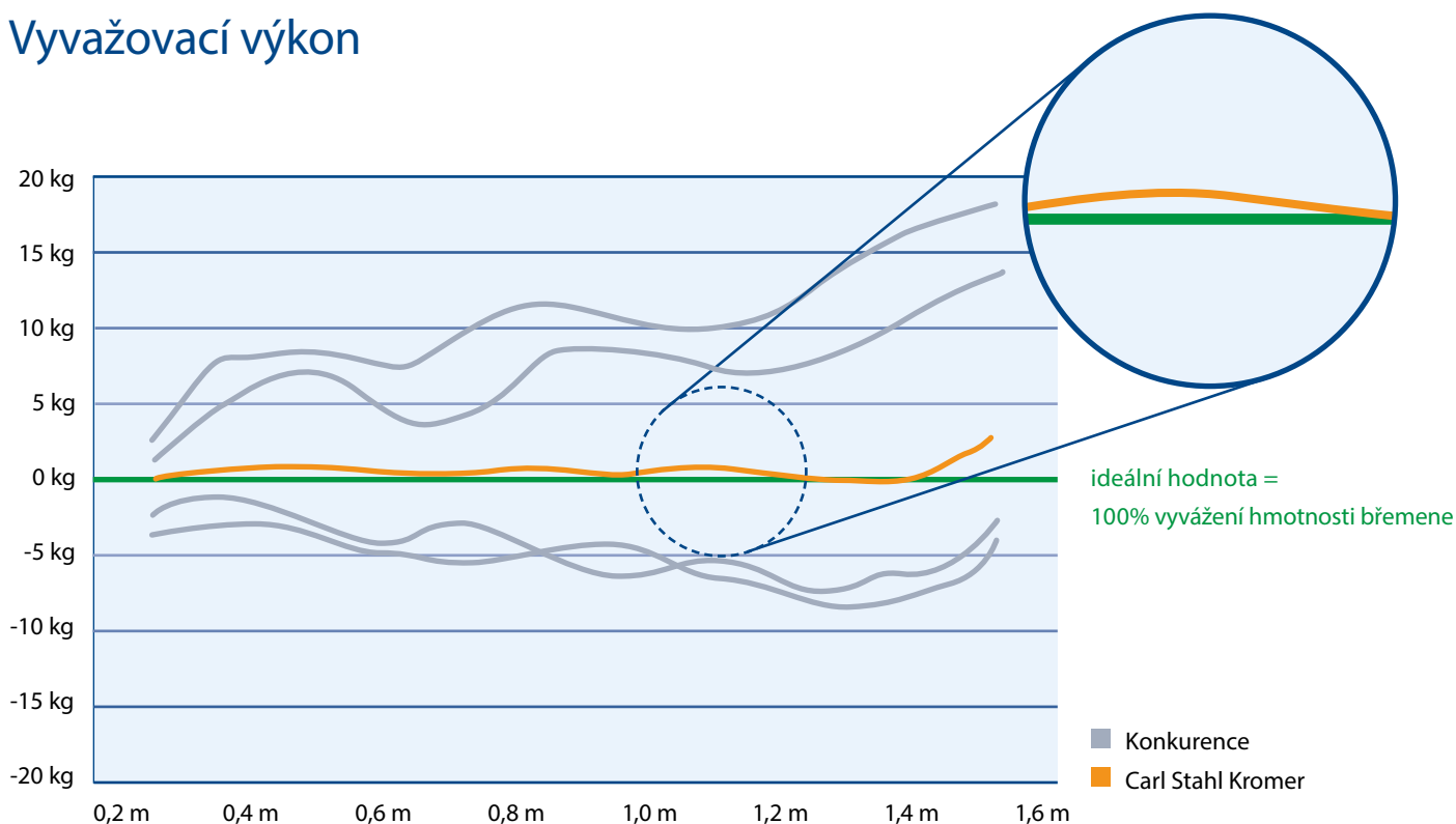
Porovnání schopnosti udržet úroveň vyvážení 85kg břemene při vysunutí 1,5 m lanka
