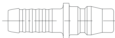
Profil spojky (originální velikost)
